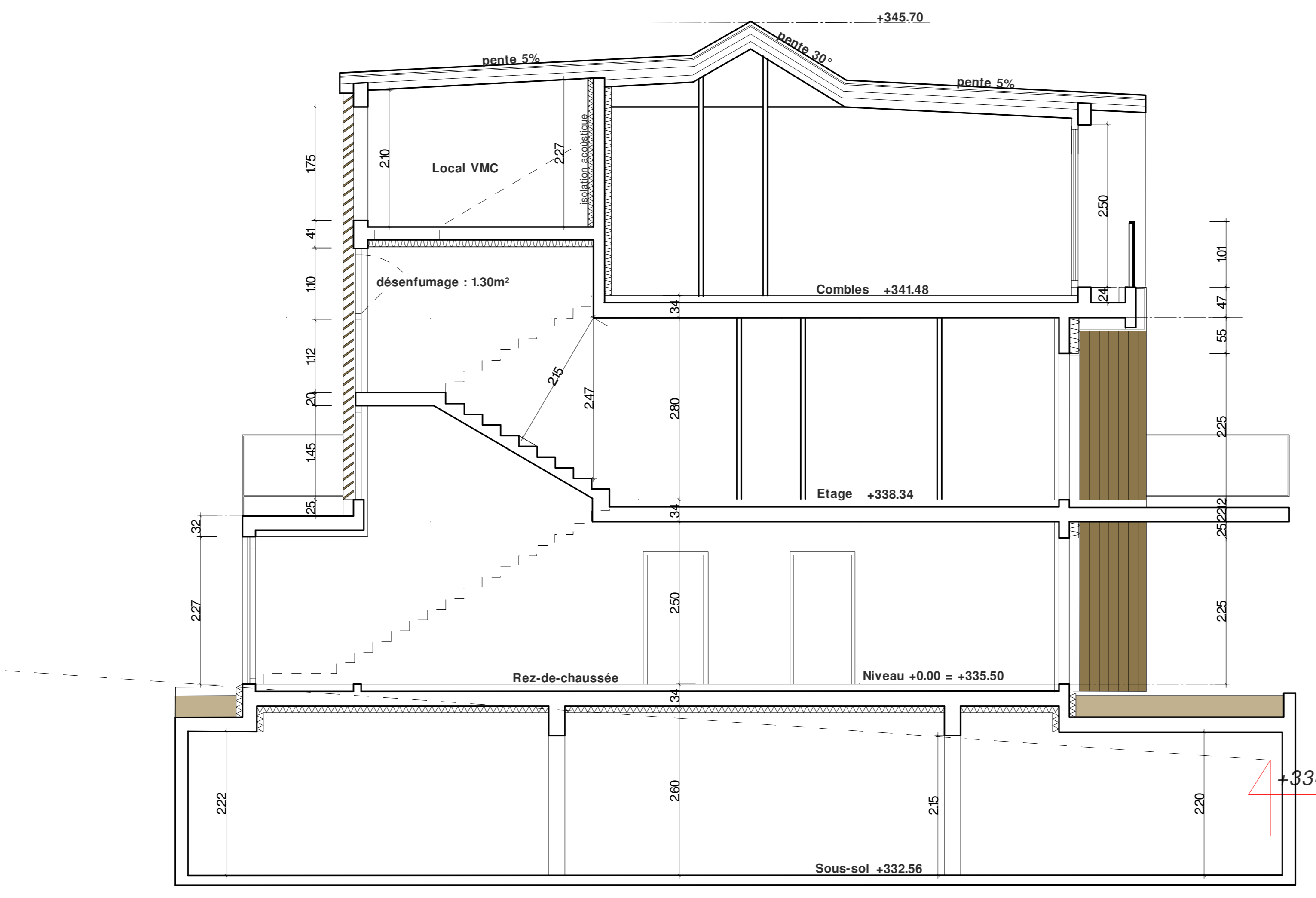
Coupe sur le bâtiment B
