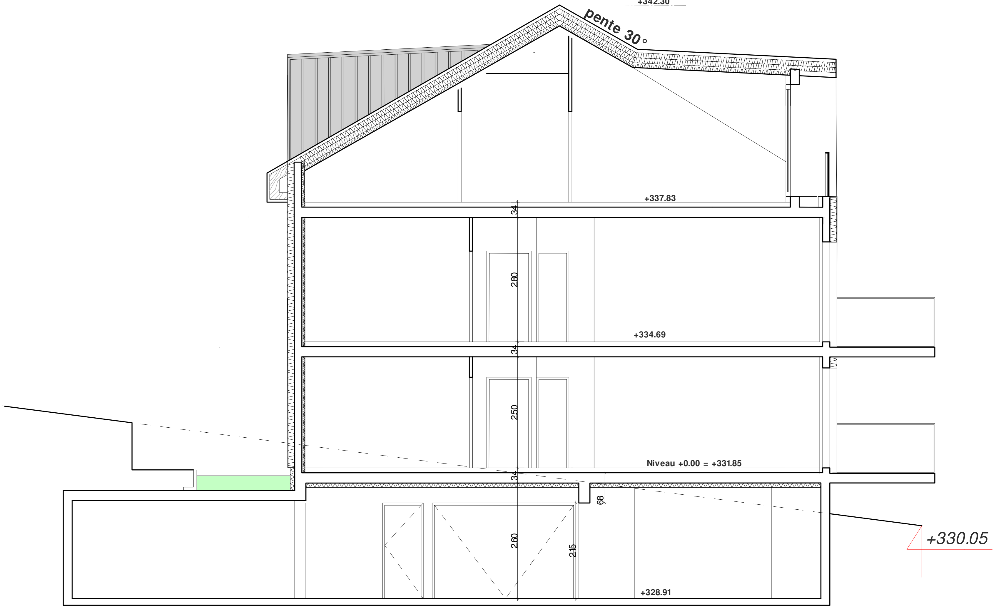
Coupe sur le bâtiment C
